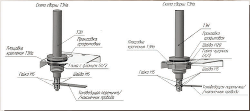
Рис.1. Вариант установки ТЭНа в парогенераторе.
