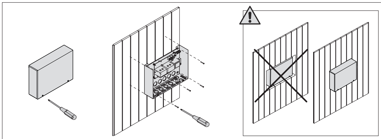
Figure 3. Ouverture du cache du bloc d'alimentation et fixations murales
