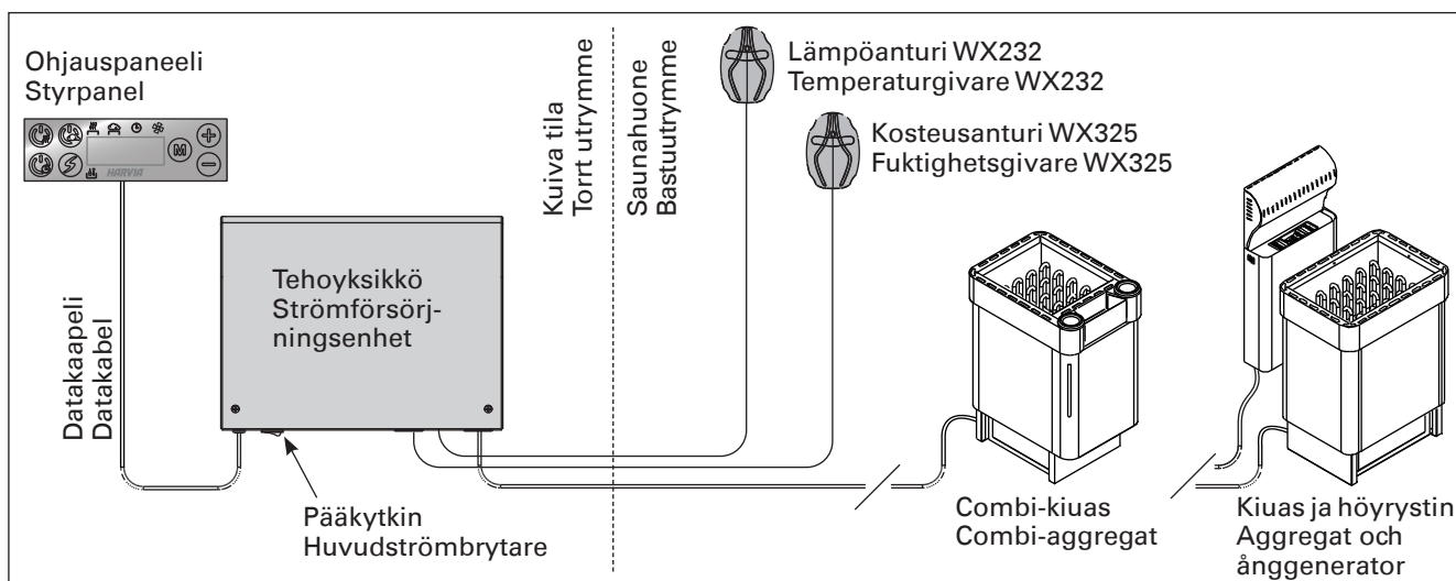
Kuva 1. Järjestelmän osat
