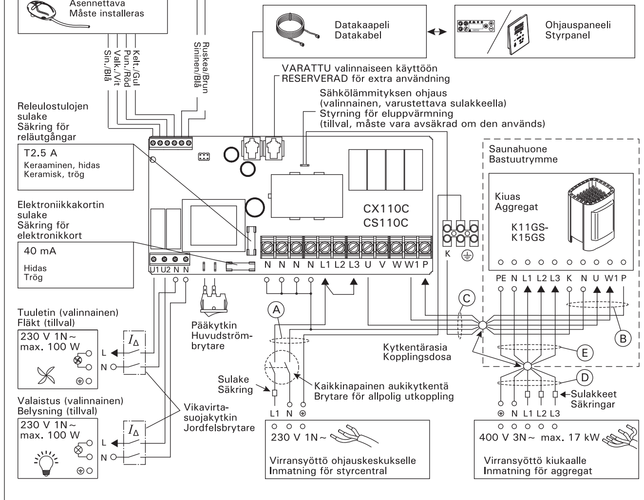
Kuva 4. Sähkökytkennät (K11GS–K15GS) Bild 4. Elektriska anslutningar (K11GS–K15GS)
