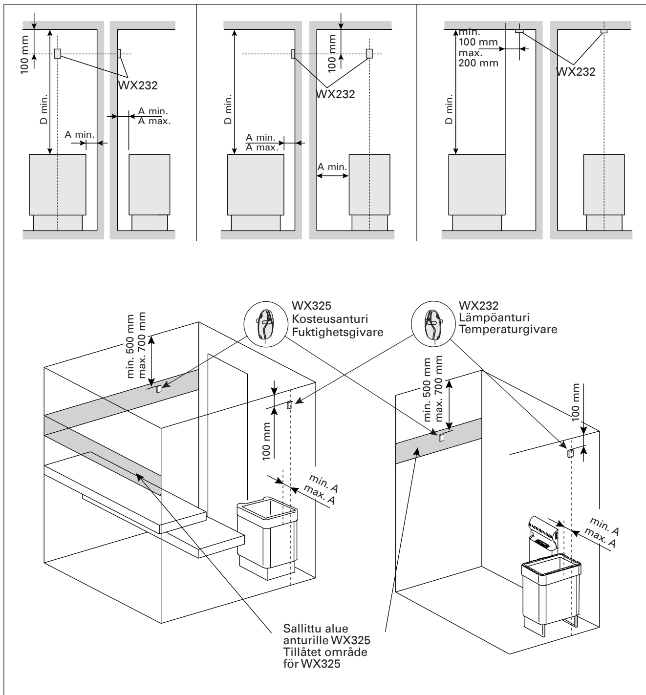
Kuva 7. Lämpö- ja kosteusantereiden sijainti lattiakiukaiden yhteydessä
