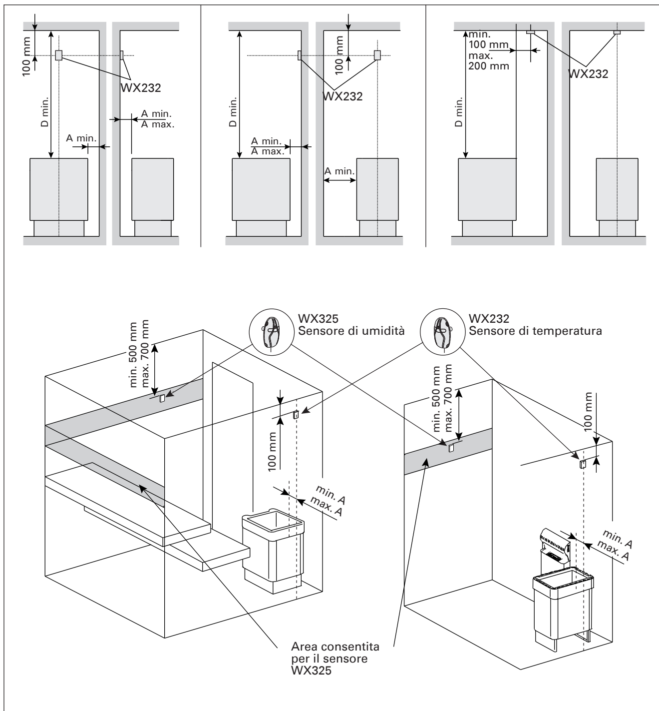
Figura 7. Posizione dei sensori di temperatura e umidità con stufe montate a pavimento
