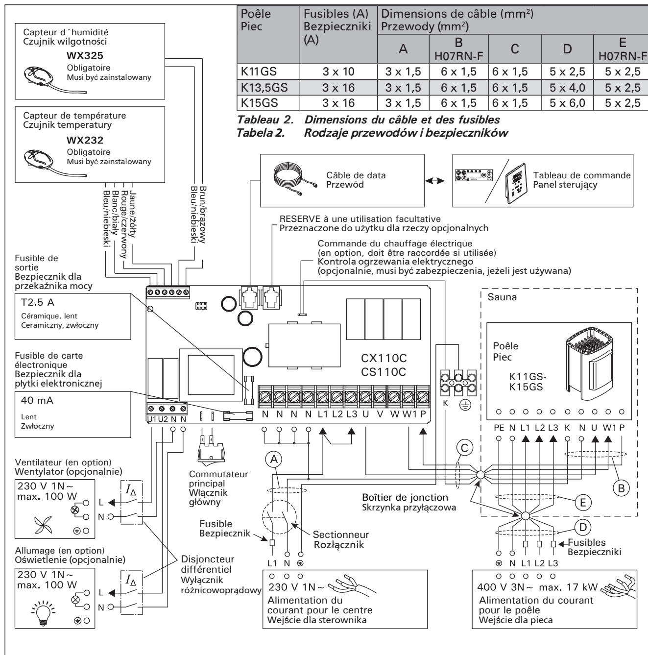
Figure 4. Raccordement électrique (K11GS-K15GS)
