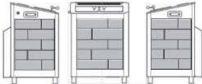
Рис. 11.1 Схема установки декоративных плит каменной облицовки для ЭНУ 10-16 кВт
