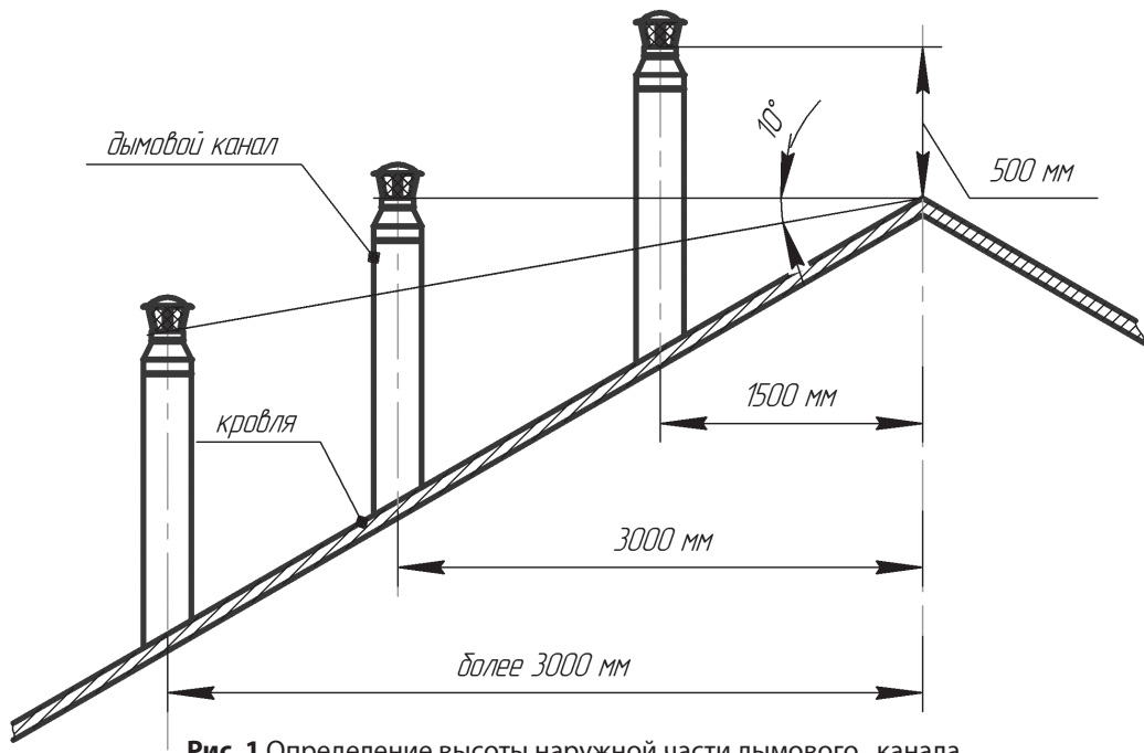
Рис. 1 Определение высоты наружной части дымового канала.
