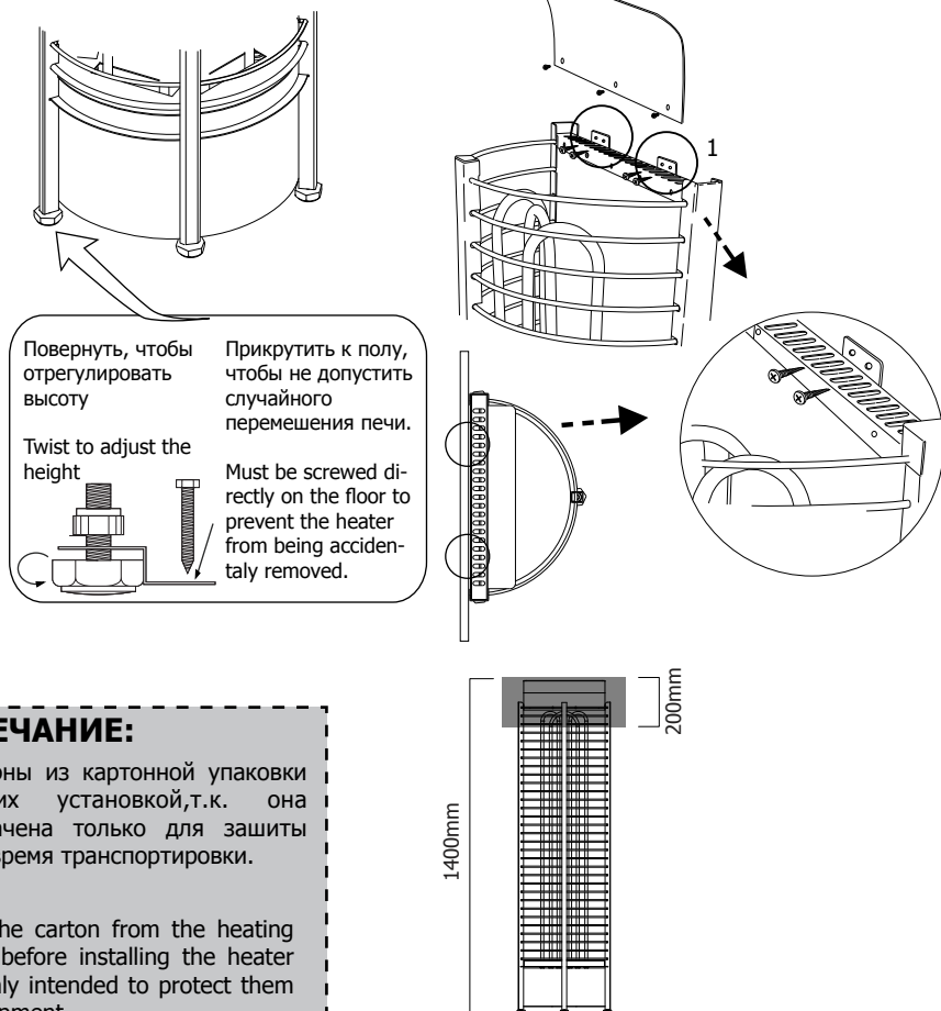
Рис. 1а. ПОДСТАВКА Fig. 1a Stand
