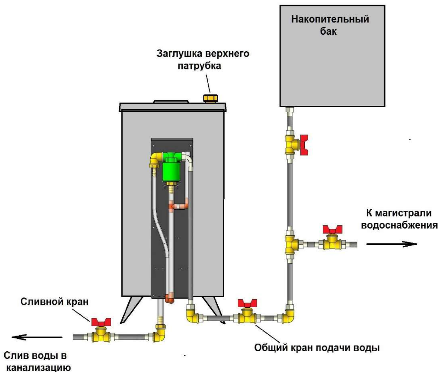
Рис.1 Типовая схема подключения ЭГПП при эксплуатации в автоматическом режиме заполнения водой.
