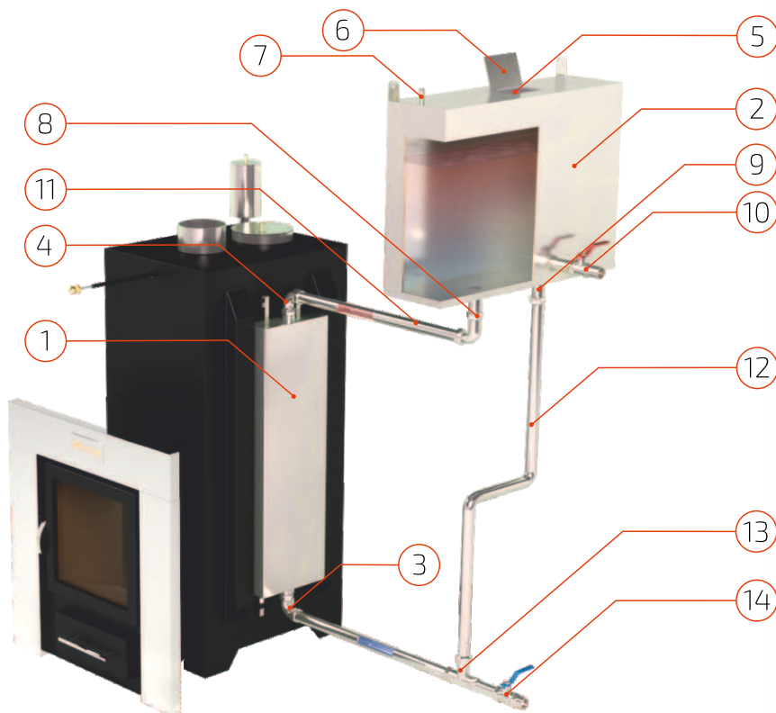
Рис. 12 Основные элементы системы подготовки горячей воды
